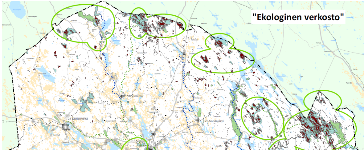
Kuva 23. Paksuturpeiset ja ojittamattomat suoalueet näkyvät kartassa ruskeina alueina. Iso osa niistä sijoittuu maakuntakaavassa osoitetuille luonnon ydinalueille (vihreä yhtenäinen rajausviiva). Paksuturpeisia suoalueita ei osoiteta kaavaehdotuksessa, vaan aineiston hyödyntämistä tutkitaan tulevissa maakuntakaavoissa.
