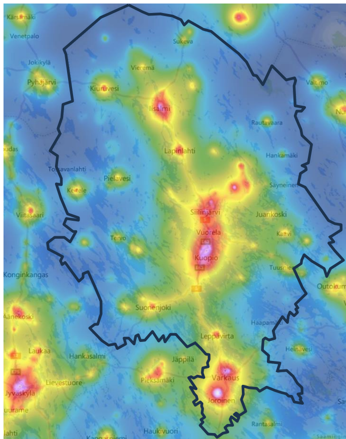
Kuva 32. Pohjois-Savon valosaaste (lähde: lightpollution map).
