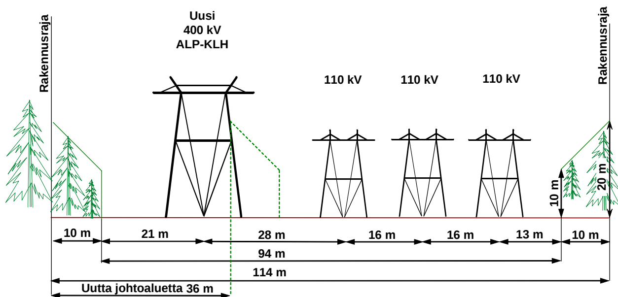
Kuva 15. Sijoituessaan kolmen 110 kV voimajohdon rinnalle uusi 400 kV voimajohto edellyttää noin 36 metriä lisää johtoaluetta. Kuva Alapitkän aseman suunnasta.
