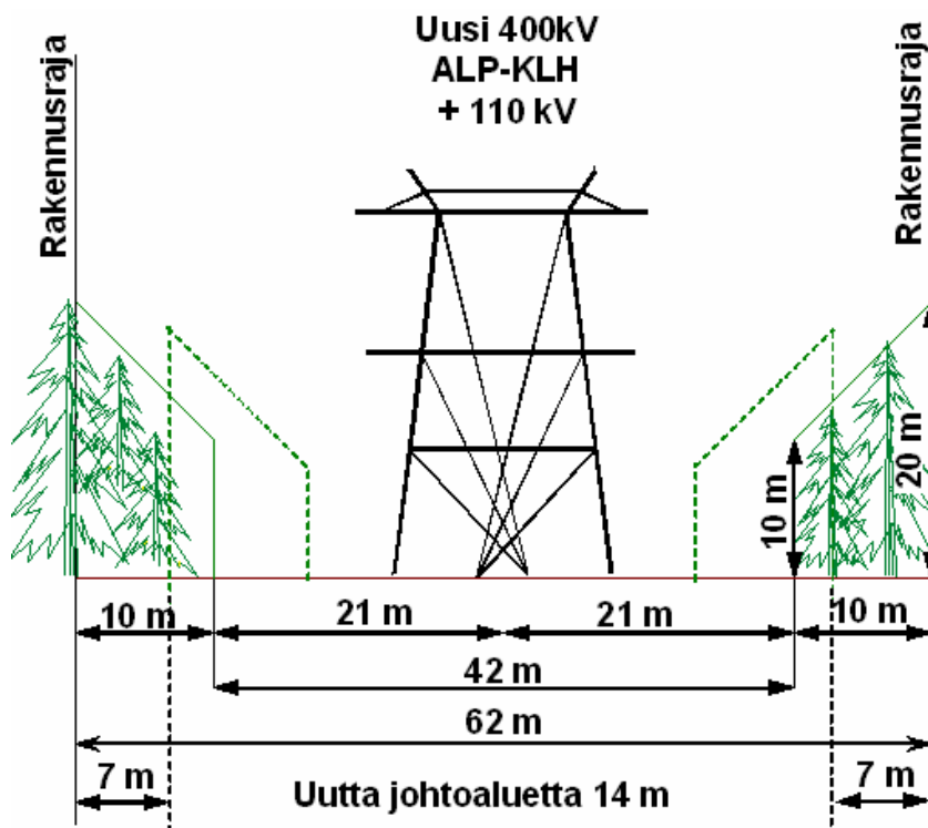
Kuva 17. Uusi 400 kV voimajohto sijoittuessaan 110 kV voimajohdon kanssa yhteispylväille edellyttää noin 14 metriä lisää johtoaluetta. Teknisesti yhteispylväs sijoitetaan nykyisen 110 kV johdon keskilinjalle. Ratkaisua käytetään ahtaissa paikoissa asutuksen läheisyydessä.
