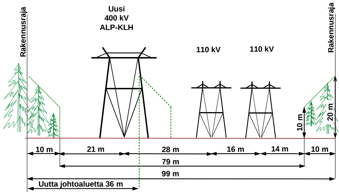
Kuva 13. Sijoituessaan kahden 110 kV voimajohdon rinnalle uusi 400 kV voimajohto edellyttää noin 36 metriä lisää johtoaluetta. Kuva Alapitkämästä Kontiolahtiin suuntaan.
