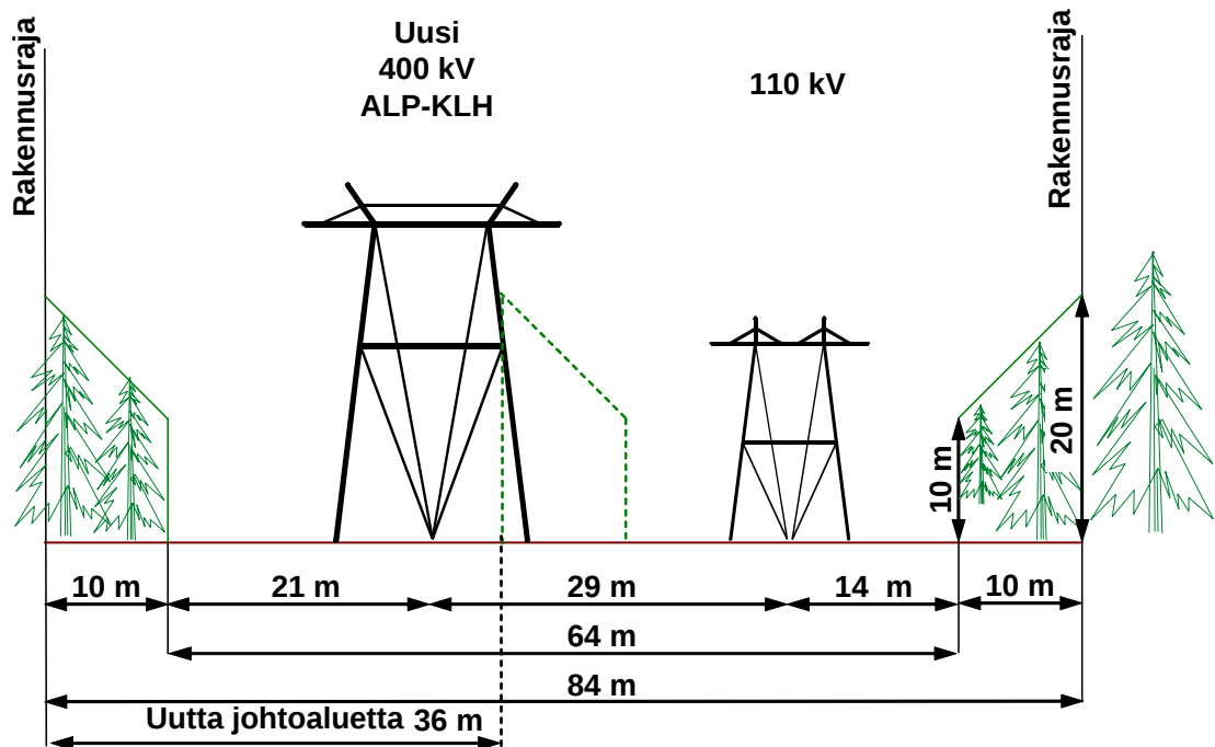
Kuva 11. Sijoituessaan 110 kV voimajohdon rinnalle uusi 400 kV voimajohto edellyttää 36 metriä lisää johtoaluetta. Kuva Alapitkäästä Kontiolahden suuntaan.
