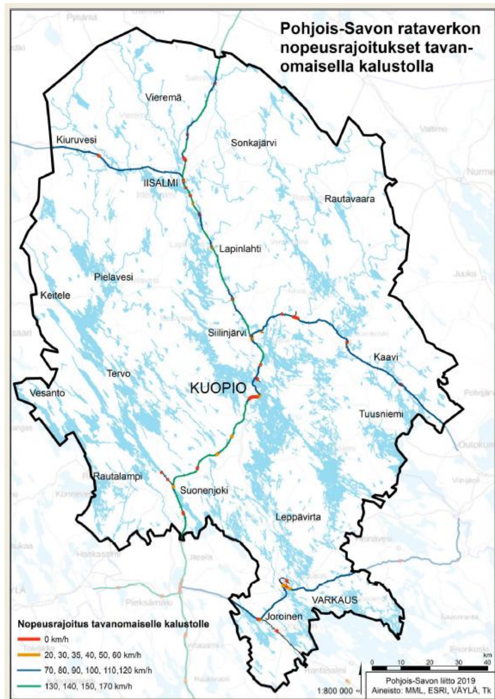
Kuva 6. Pohjois-Savon rataverkosto nopeusrajoituksineen.
